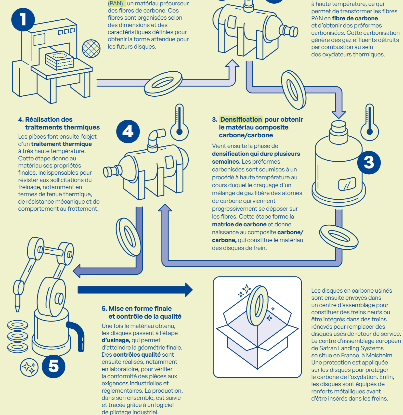
→ Schéma du processus de production du projet 4U.
